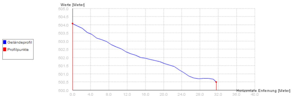
nördliches West-Ost-Geländemodell
